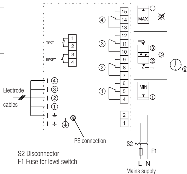
Fig. 2 Wiring diagram
